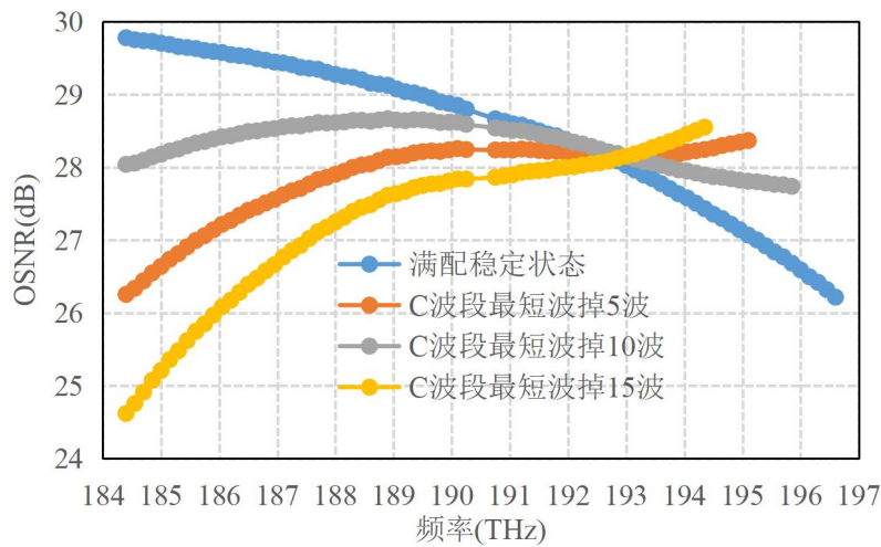
图3.5. C+L掉波场景性能验证
