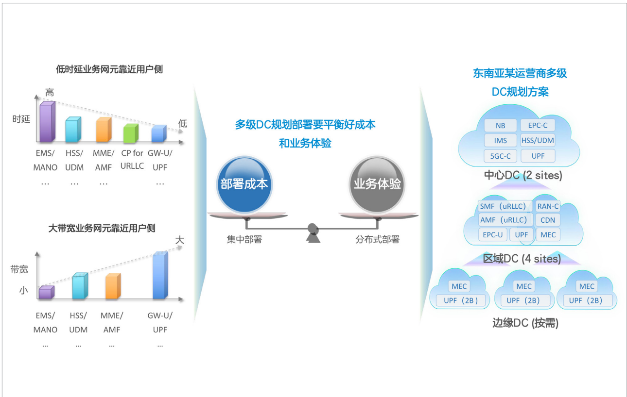
图 4 多级 DC 部署规划
