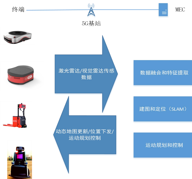
图 4-8 5G+SLAM 定位方案
