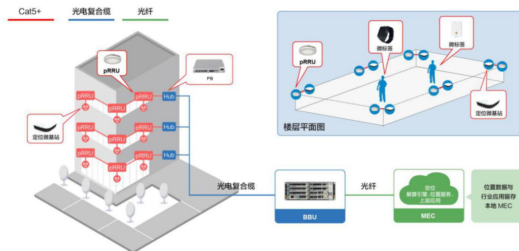
图 4-5 5G 融合 UWB/蓝牙 AOA 组网架构
