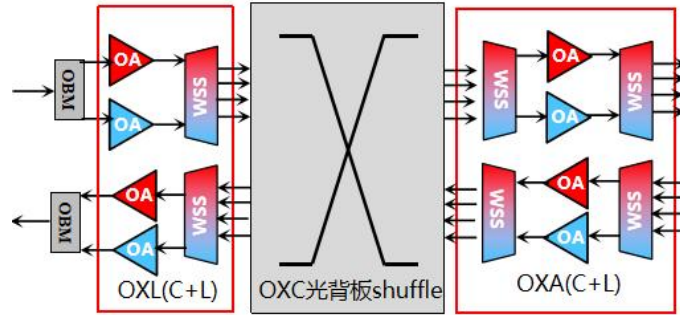
图 2.7 C+L WSS 一体化 OXC 架构
