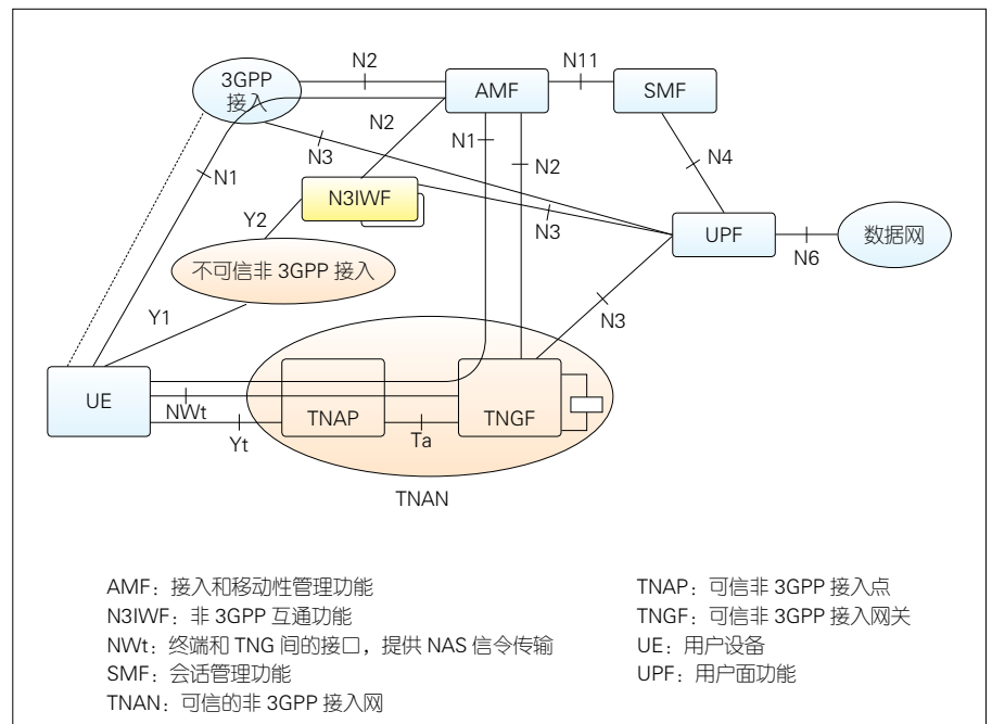
▲图 1 可信及非可信非 3GPP 接入架构
