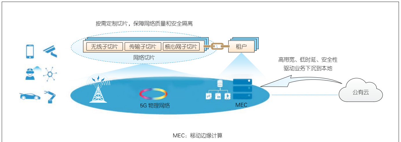
▲图3 切片与 MEC 协同构建行业一体化服务
