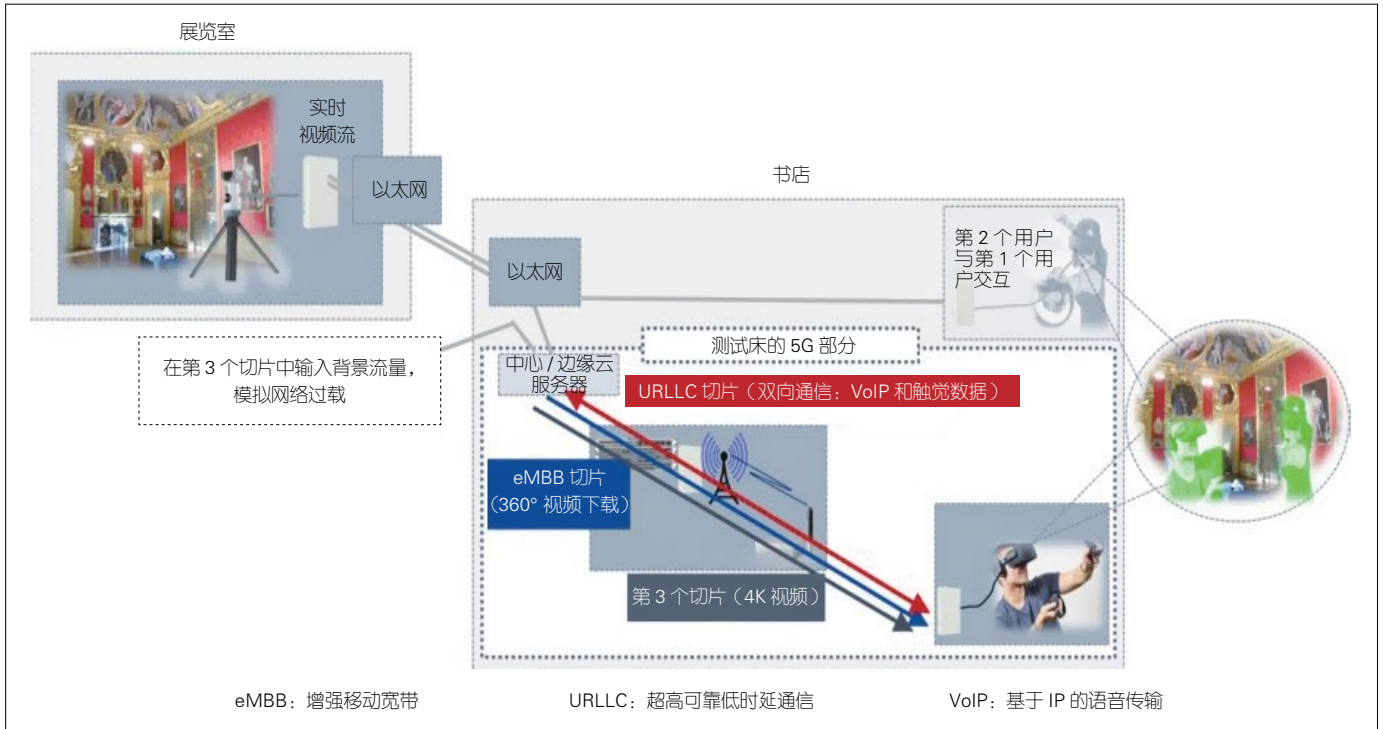
▲图 3 网络人工智能标准工作组系统辅助的弹性网络切片管理测试床 [2]
