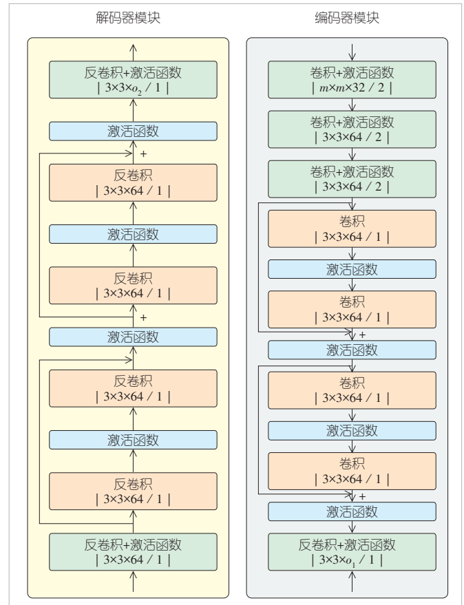
▲图3 编码器模块、解码器模块结构示意图
