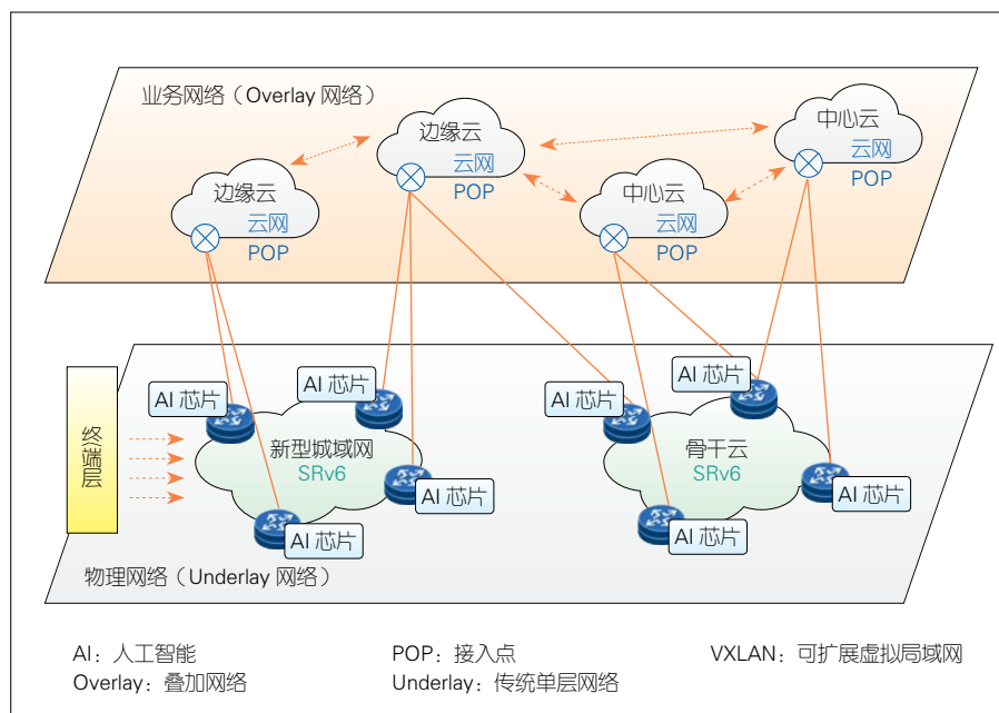
▲图 4 结合 Underlay 和 Overlay 的弹性组网模式
