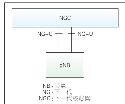
▲图3 Option 2架构
