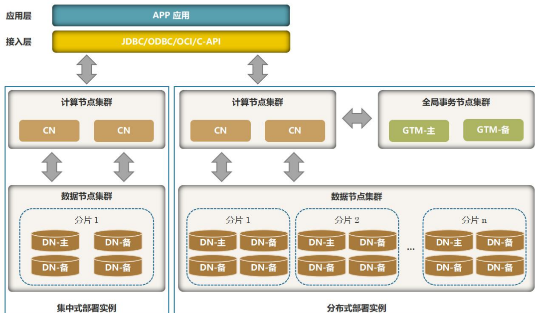
图 3.2-3 混合部署
