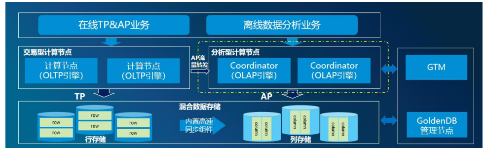
图 3.1-4 GoldenDB HTAP 架构
