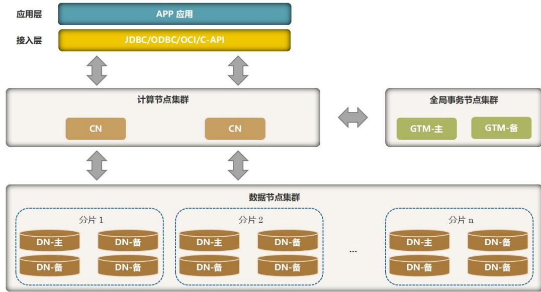
图 3.2-2 分布式部署
