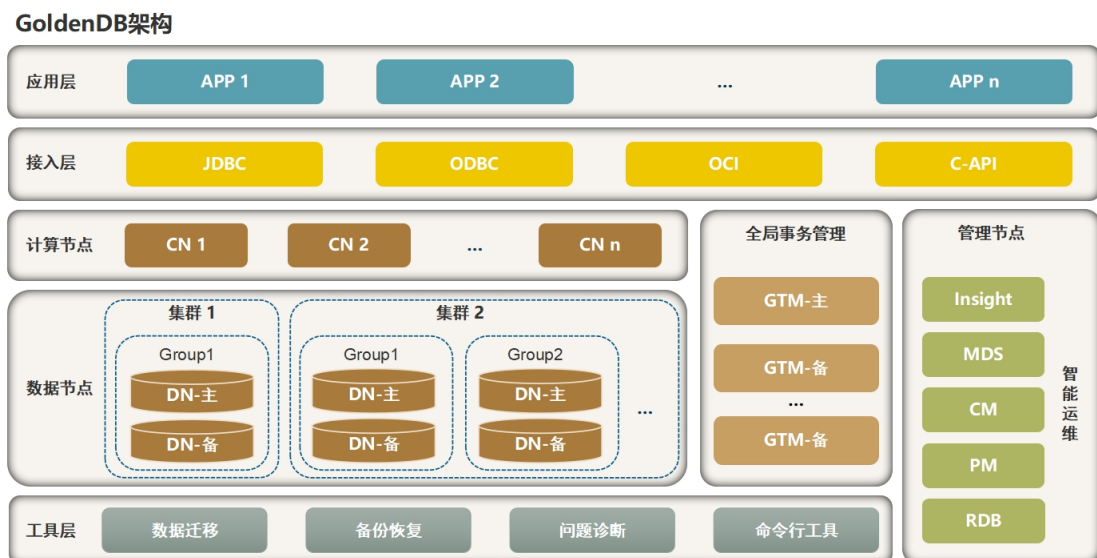
图 3.1-1 GoldenDB 逻辑架构图
