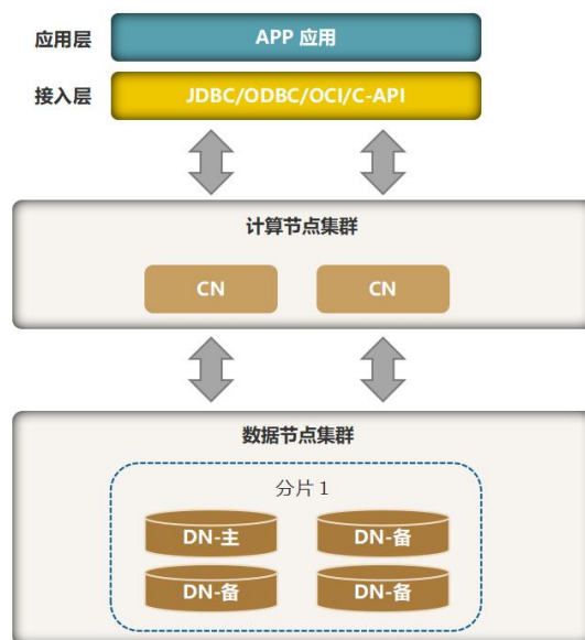
图 3.2-1 集中式部署
