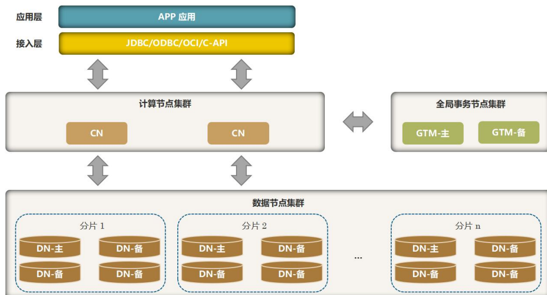
图 3.2-2 分布式部署
