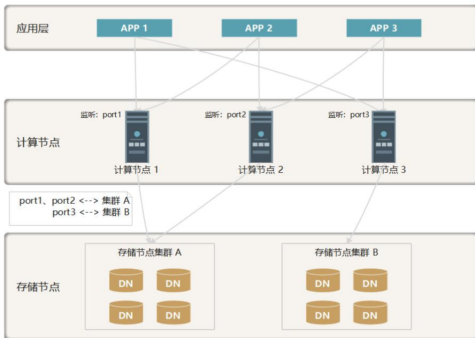
图 3.1-2 应用访问关系图
