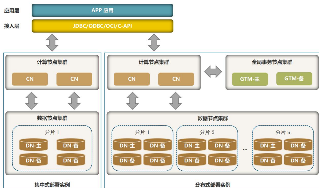
图 3.2-3 混合部署
