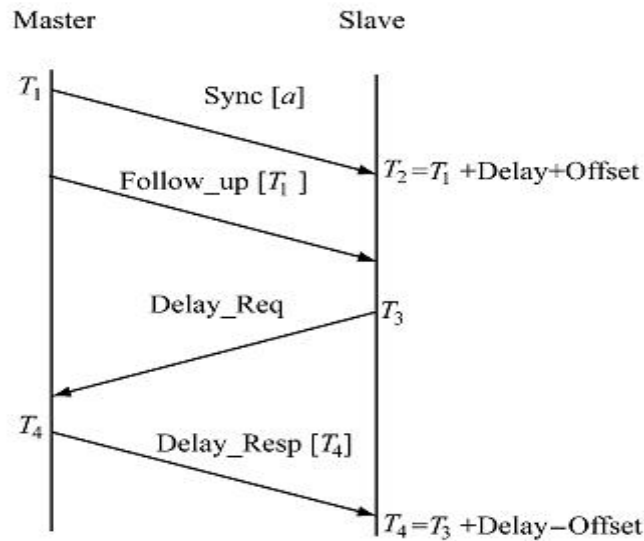
图 12 1588 的协议实现
