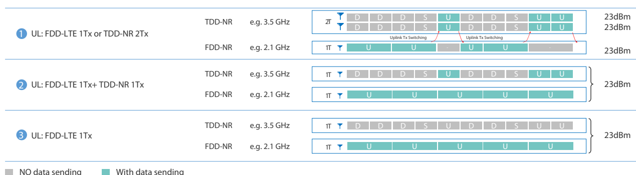
图 支持 Uplink Tx Switching (CA) 的终端上行工作模式
