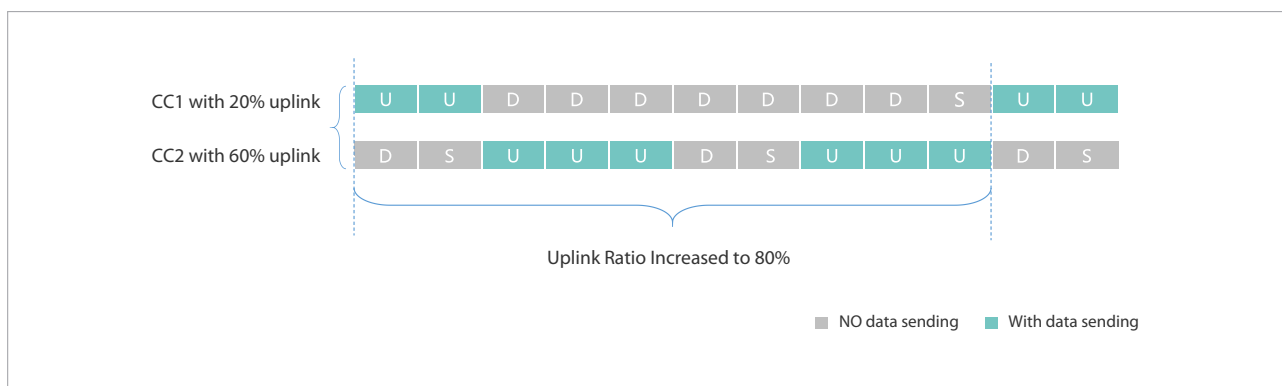
图 两个 TDD 异帧情况下采用 CA 后的终端工作模式
