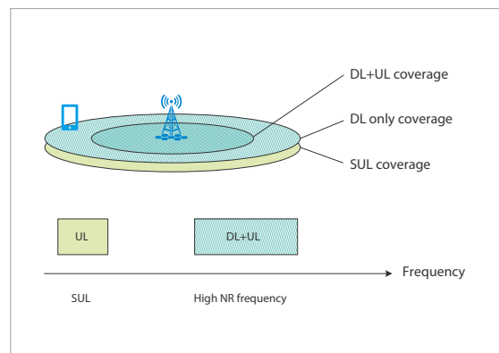
图 SUL 示意图
