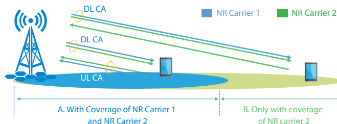
图 UL CA (Inter-Band) 的应用场景
