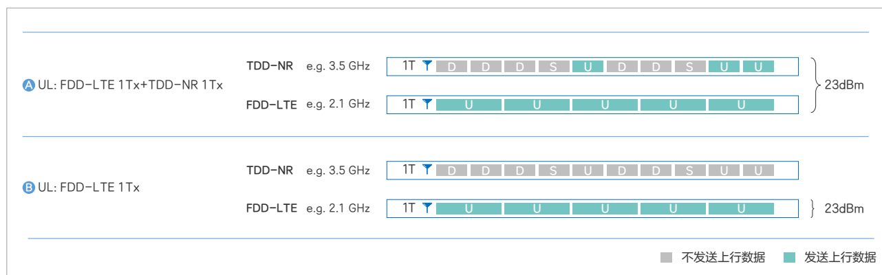
图 EN-DC 架构下终端上行工作模式
