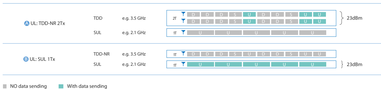
图 SUL 的终端上行工作模式
